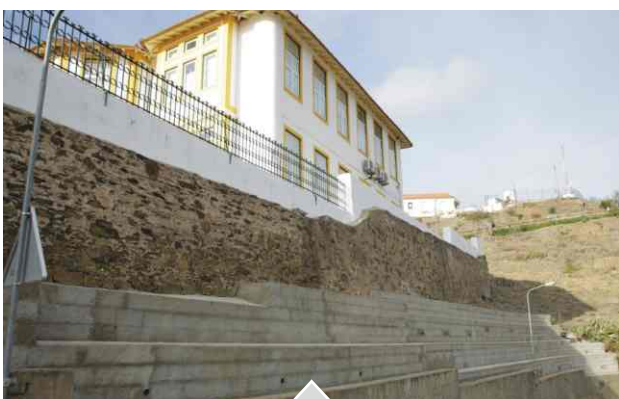
// Reforço de Muro Escola Primária, Mértola
